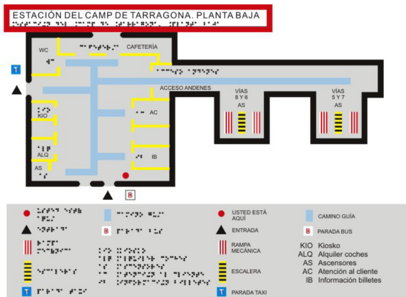
Imagen 6. Ubicación del título en un plano horizontal
